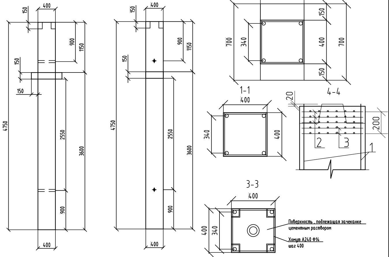
Колонна К-1
