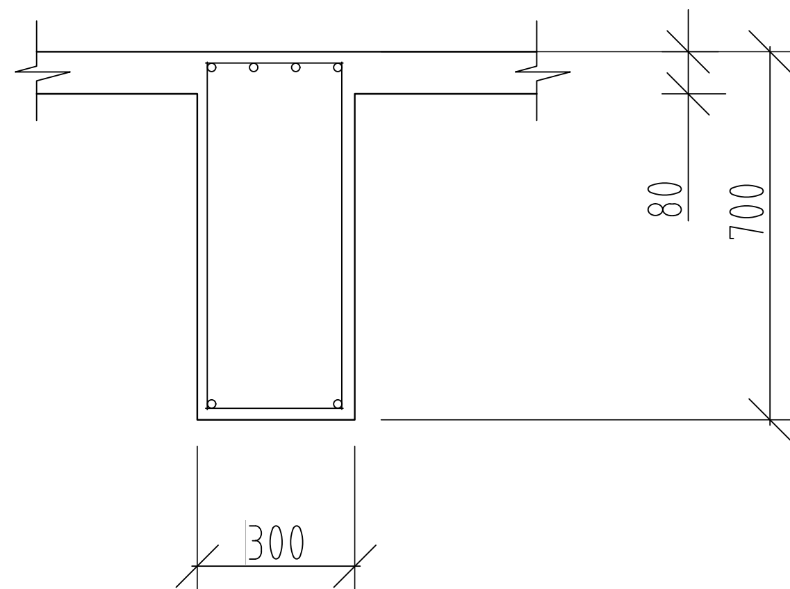
Разрез 4-4
