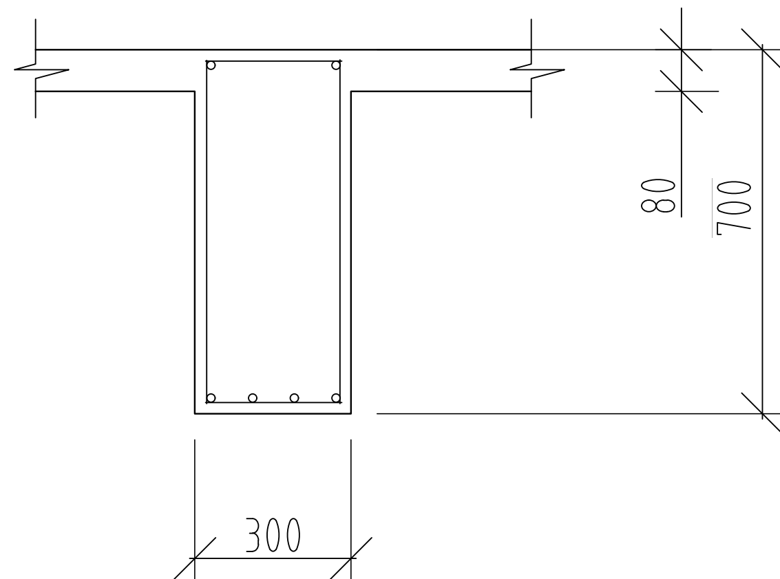
Разрез 3-3
