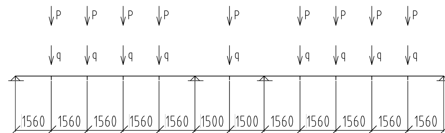
Расчетная схема
