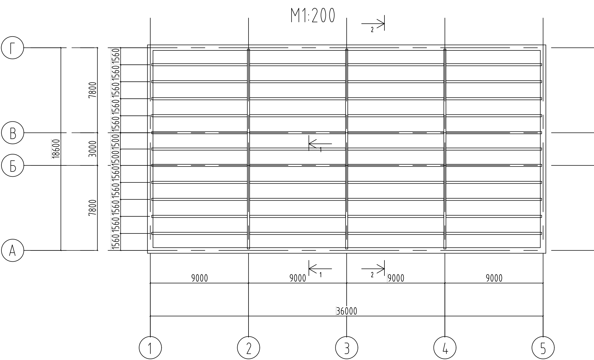
Схема расположения главных и второстепенных балок
