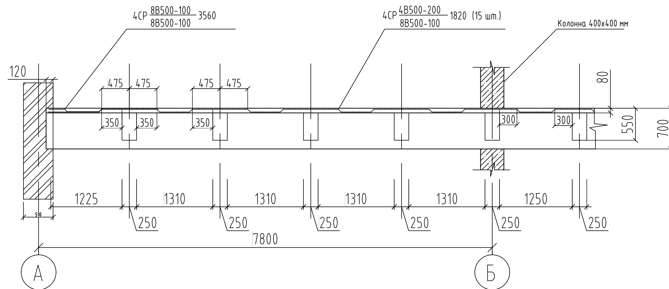
Расчетная схема
