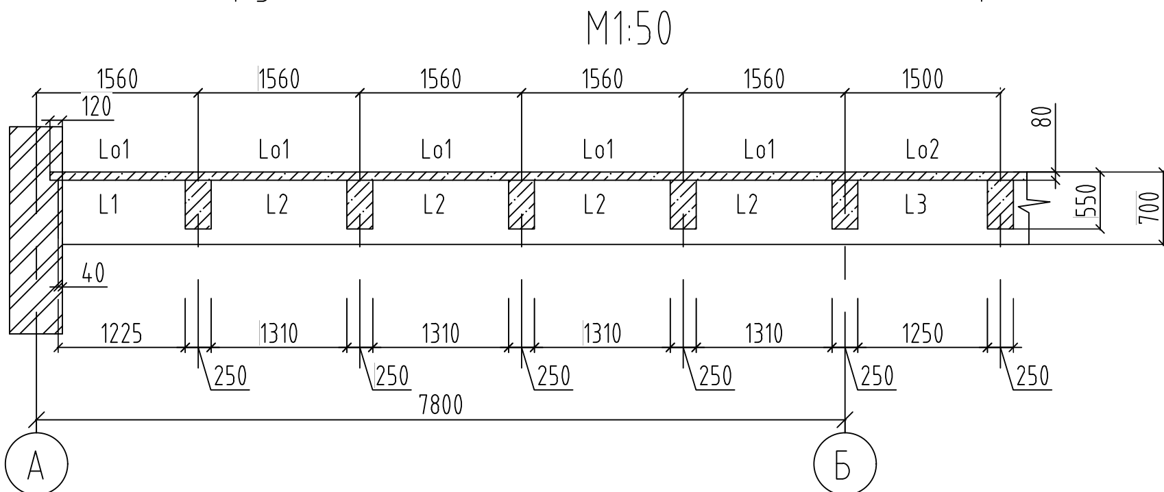
Конструктивная схема монолитной плиты (Разрез 1-1)
