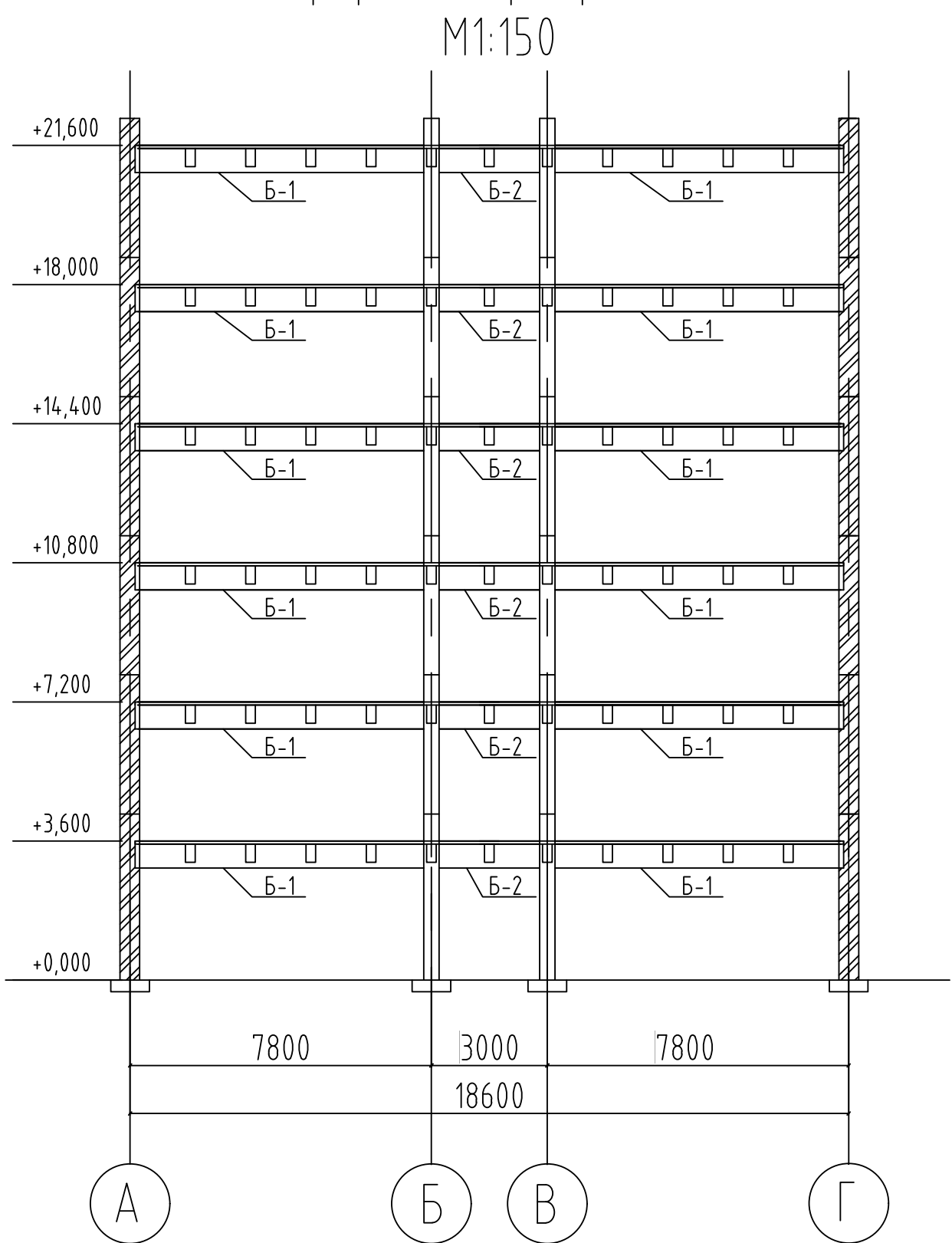
Конструктивная схема монолитной плиты (Разрез 1-1)
