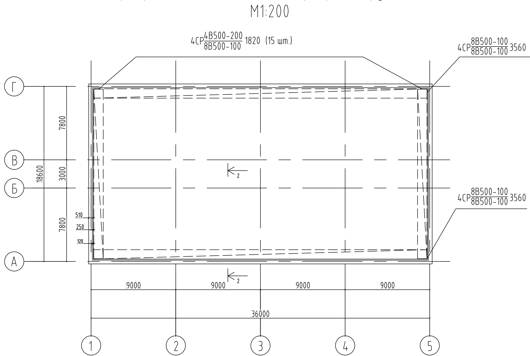
Схема армирования монолитного перекрытия рулонными сетками
