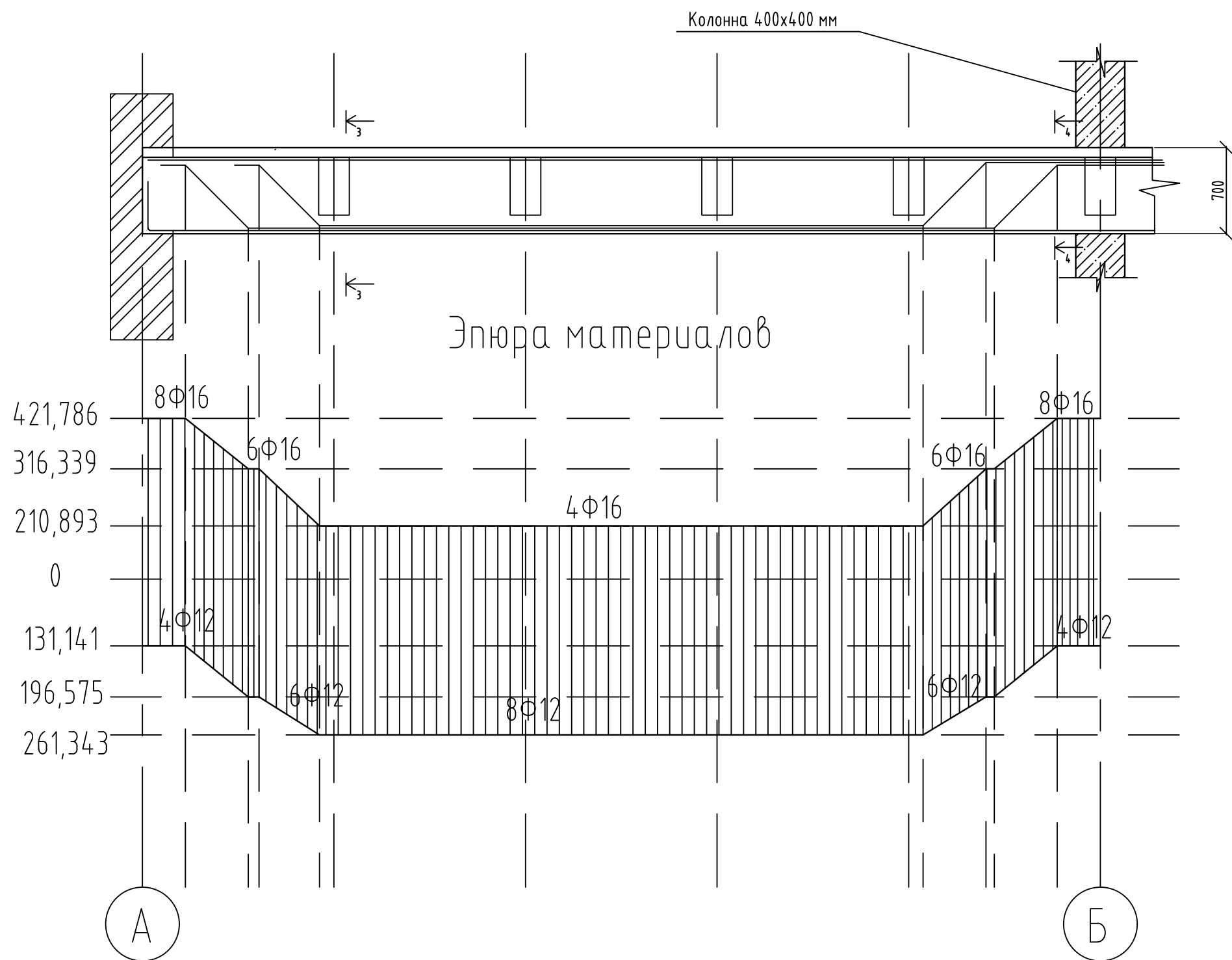
Схема армирования Б1 М1:40
